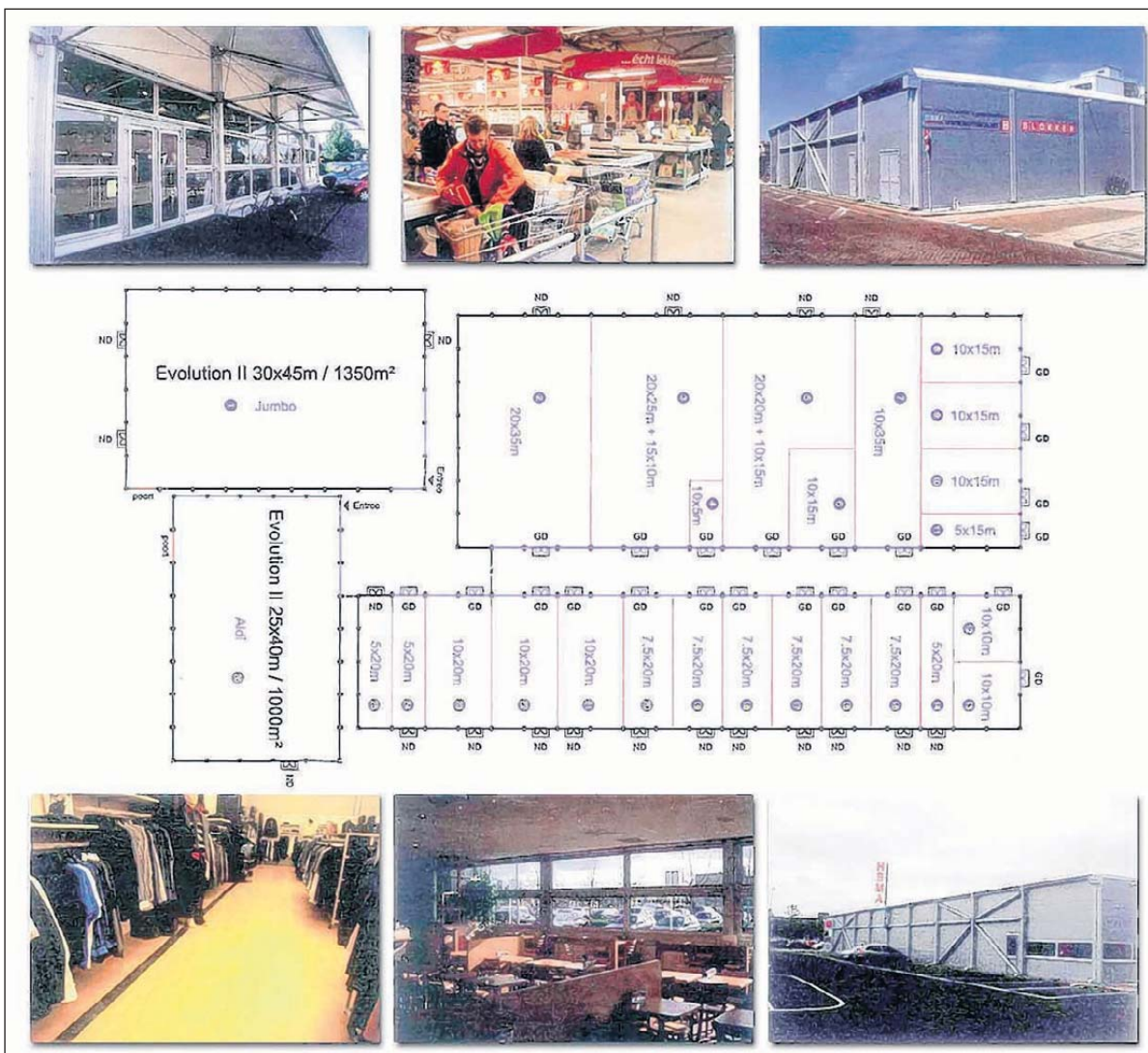
Indeling tijdelijke winkelvoorziening Omphaliusplein en voorbeelden constructie en interieur. illustratie Neptunus
